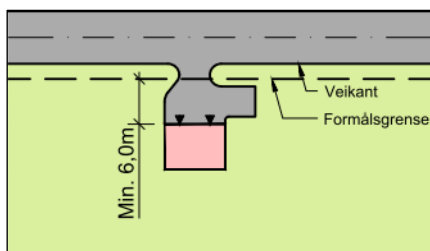
Figur 5.7: Garasje, vinkelrett på vei
