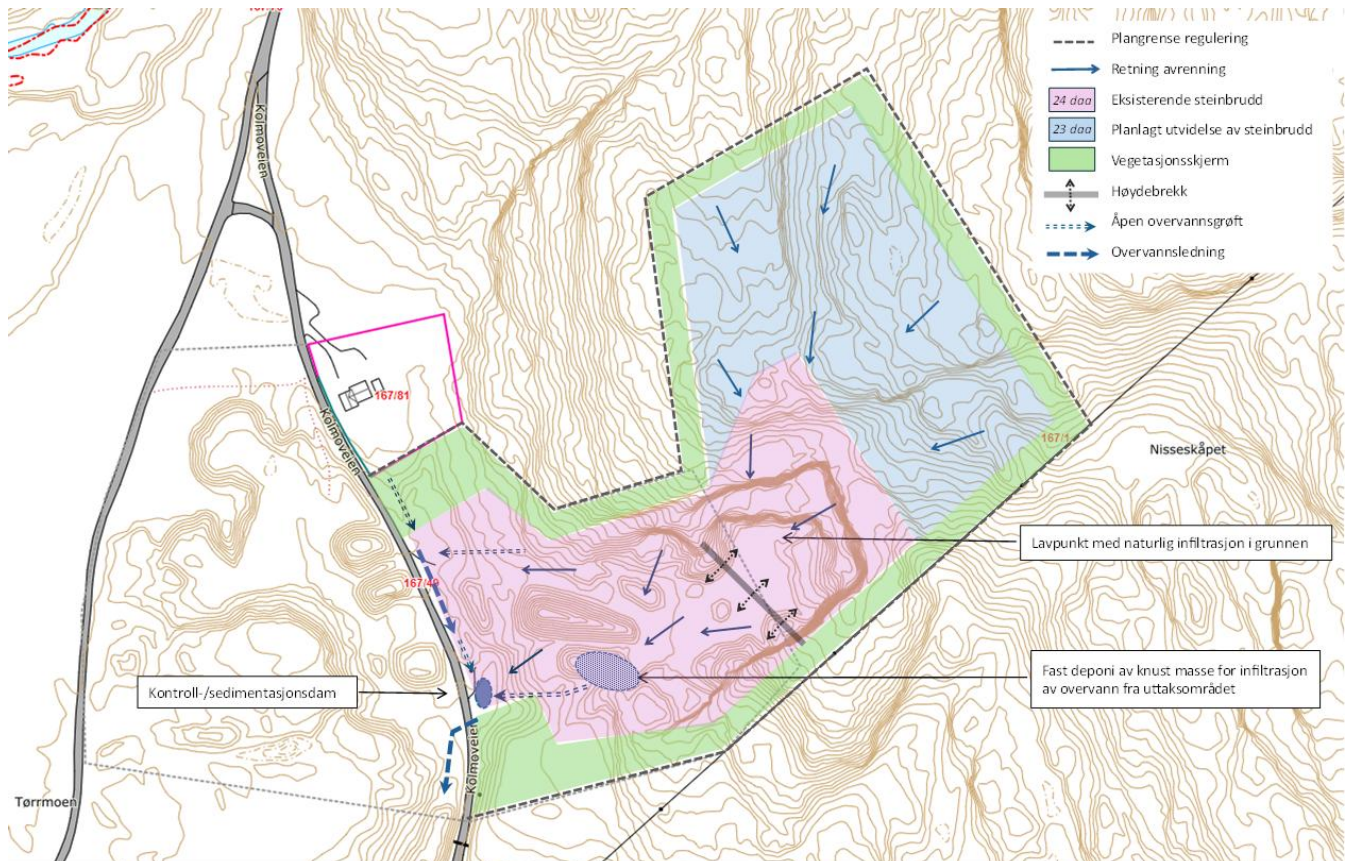
Figur 12: Overvannsplan (vedlegg 8)
