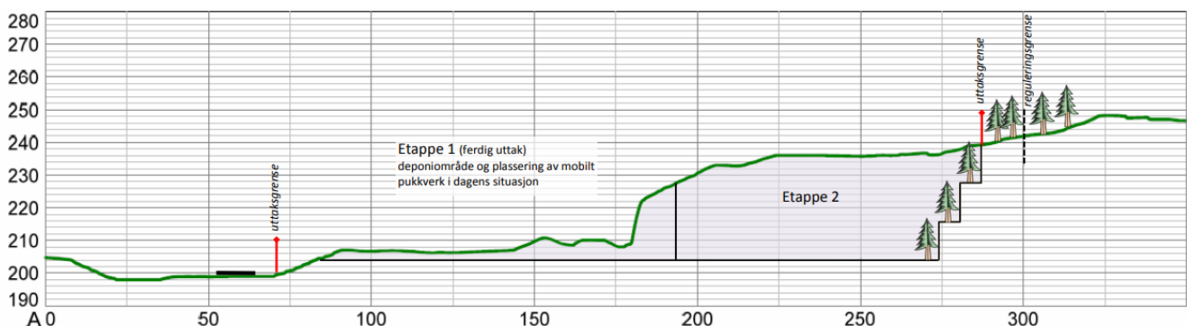
Figur 7: illustrasjonssnitt øst-vest i eksisterende uttaksområde (Driftskonsesjon for Tørrmoen masseuttak, 17.09.19)
